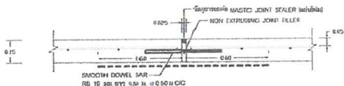
ขยายรอยต่อ EXPANSION JOINT ทุกระยะ 50 เมตร
