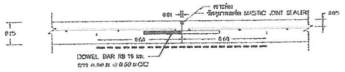
ขยายรอยต่อ CONSTRUCTION JOINT ทุกระยะ 10 เมตร SCALE _____ NOT
