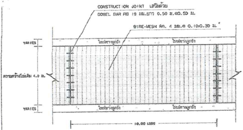
รูปแปลนผิวจราจรคอนกรีตเสริมเหล็ก SCALE _____ NOT
