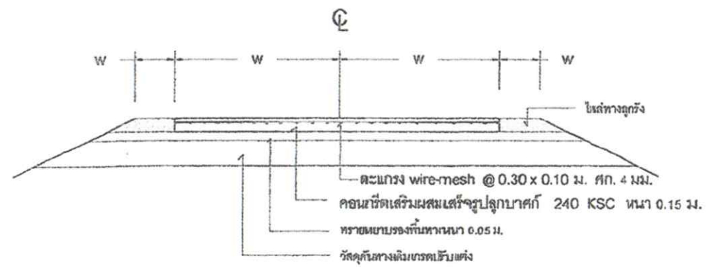
รูปตัดถนนคอนกรีตเสริมเหล็ก SCALE _____ NOT
