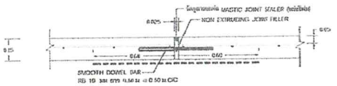
ขยายรอยต่อ EXPANSION JOINT ทุกระยะ 50 เมตร SCALE _____ NOT
