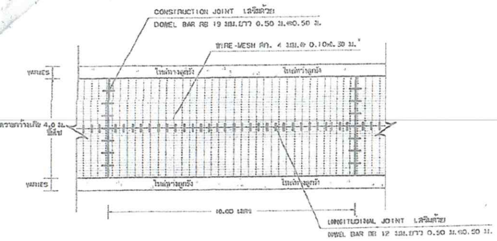
รูปแปลนผิวทางคอนกรีตเสริมเหล็ก SCALE: NOT
