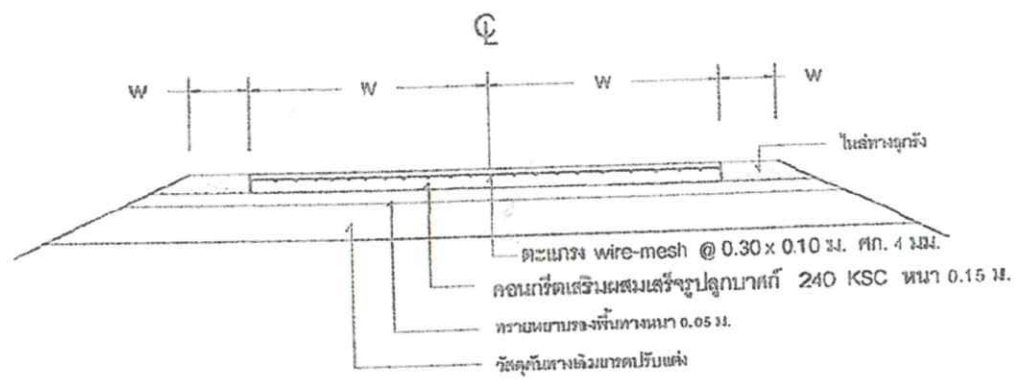
รูปตัดถนนคอนกรีตเสริมเหล็ก SCALE: NOT
