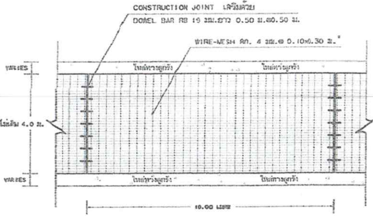
รูปแบบผิวจราจรคอนกรีตเสริมเหล็ก SCALE _____ NOT
