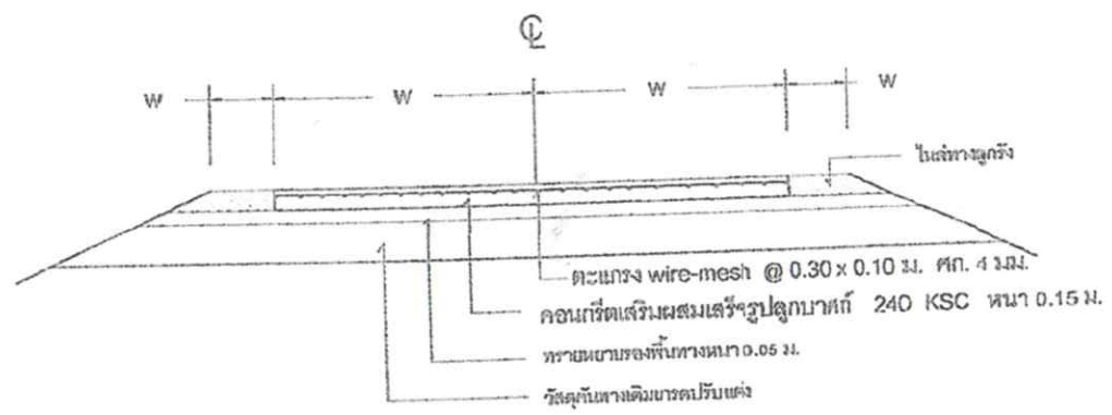
รูปตัดตามคอนกรีตเสริมเหล็ก SCALE 1:10
