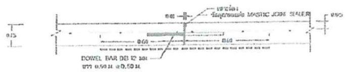
รอยต่อตามยาว (LONGITUDINAL JOINT) SCALE 1:10
