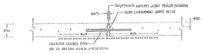
ขยายรอยต่อ EXPANSION JOINT ทุกระยะ 50 เมตร SCALE 1:10
