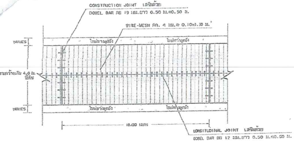
รูปแปลนผิวจราจรคอนกรีตเสริมเหล็ก SCALE 1:100
