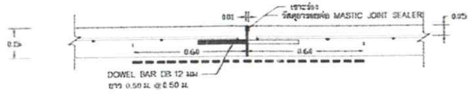
รอยต่อตามยาว (LONGITUDINAL JOINT) SCALE _____ NOT
