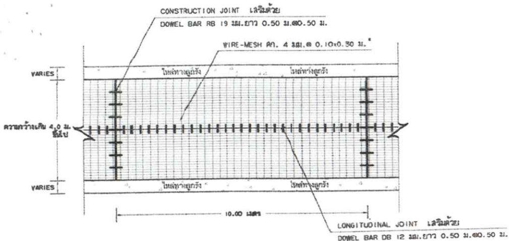
รูปแปลนผิวจราจรคอนกรีตเสริมเหล็ก SCALE _____ NOT
