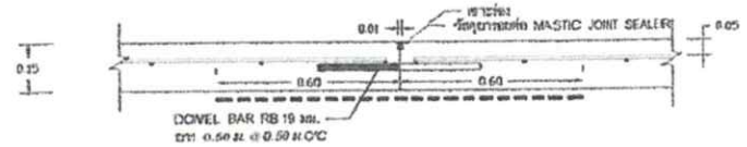
ขยายรอยต่อ CONSTRUCTION JOINT ทุกระยะ 10 เมตร SCALE _____ NOT
