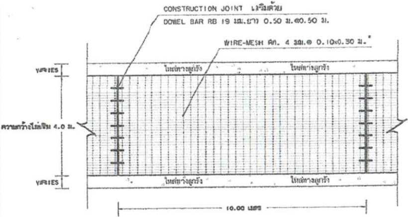
รูปแปลนผิวจราจรคอนกรีตเสริมเหล็ก SCALE _____ NOT
