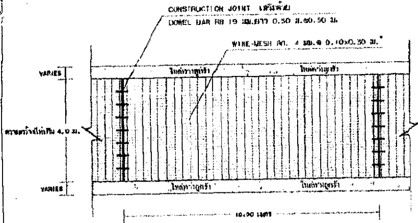
รูปแปลนผิววางวางคอนกรีตเสริมเหล็ก SCALE: NOT
