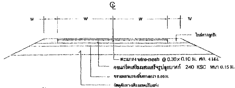
รูปตัดตามแนวของคอนกรีตเสริมเหล็ก SCALE: NOT
