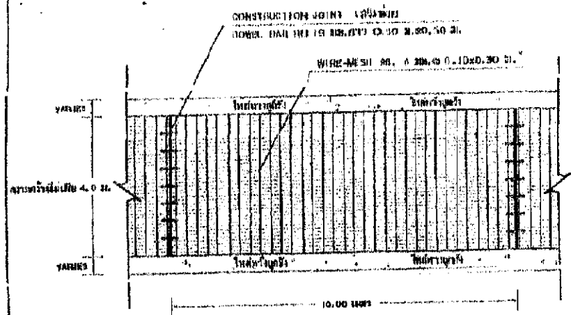
รูปแบบผิวหน้าของคอนกรีตในเขตรอยต่อ SCALE: 1:10
