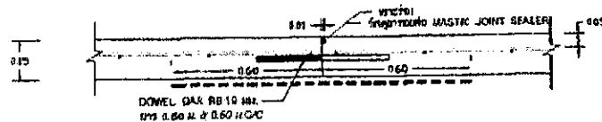
ขยายรอยต่อ CONSTRUCTION JOINT ทุกระยะ 10 เมตร
