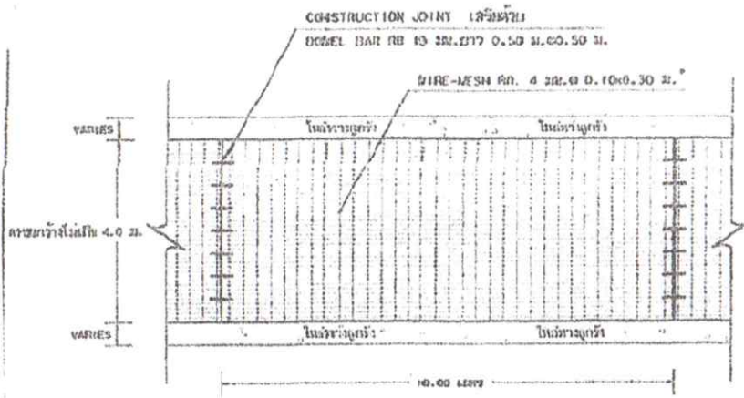
รูปแบบลงมือวางวางคอนกรีตเสริมเหล็ก SCALE: NOT
