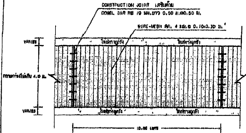
รูปแปลนผิววางรอยต่อเสริมเหล็ก SCALE: NOT
