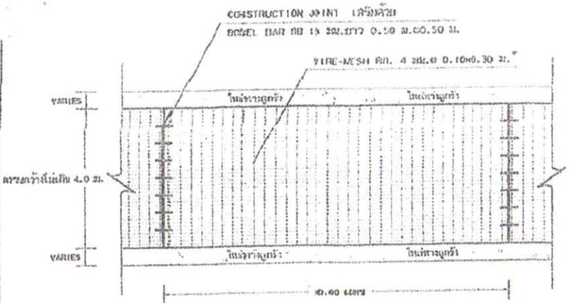
รูปแบบฉนวนคอนกรีตเทวีธอนเหล็ก SCALE: 1:100
