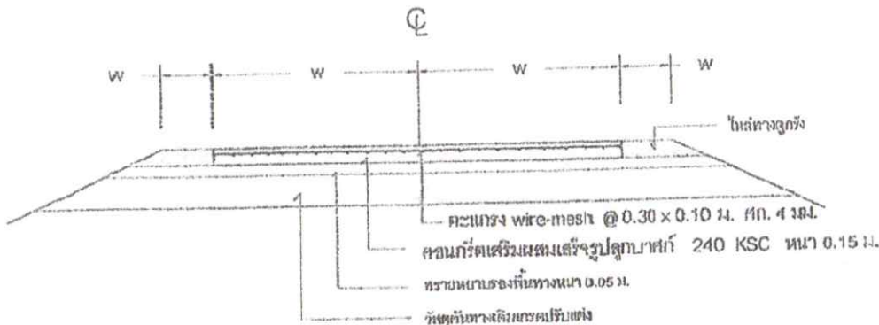
รูปแบบฉนวนคอนกรีตเทวีธอนเหล็ก SCALE: 1:100
