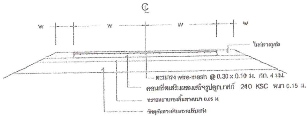
รูปตัดแนวคอนกรีตเสริมเหล็ก SCALE: NOT
