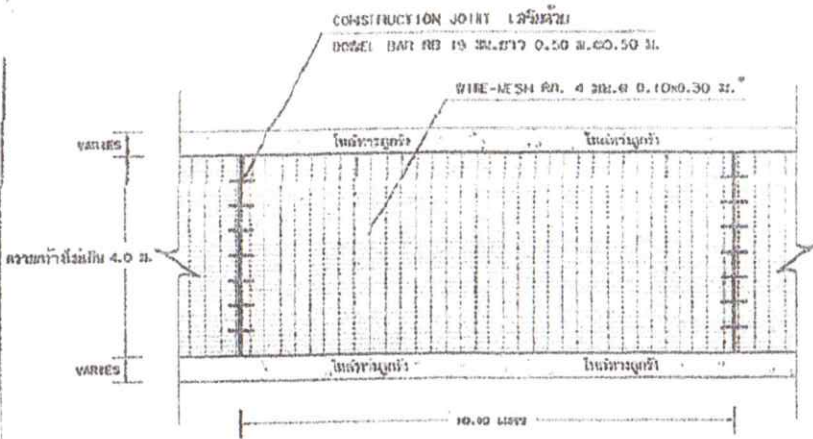
รูปแบบผิวจราจรคอนกรีตเสริมเหล็ก SCALE: NOT
