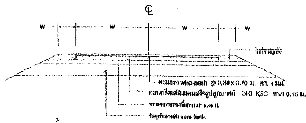
รูปตัดคอนกรีตคอนกรีตผิวหน้าเหล็ก SCALE: 1:100
