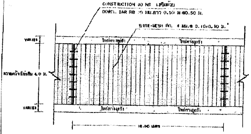
รูปแบบผิววางวางคอนกรีตเสริมเหล็ก SCALE: _____ NOT
