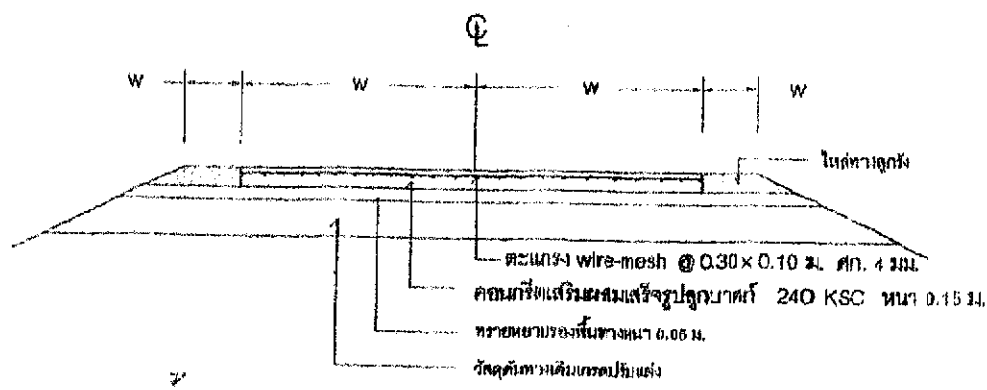
รูปตัดหน้าคอนกรีตเสริมเหล็ก SCALE: _____ NOT
