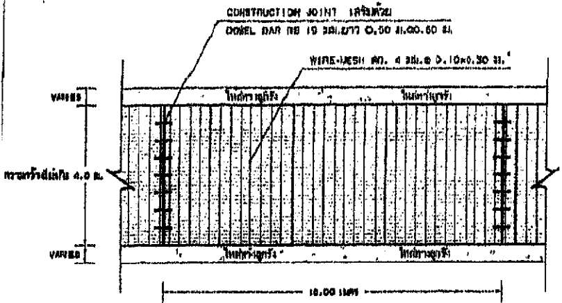
รูปแปลนผิวทางคอนกรีตเสริมเหล็ก SCALE ..... NOT
