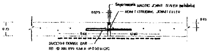
ขยายรอยต่อ EXPANSION JOINT ทุกกระยะ 50 เมตร SCALE: NOT
