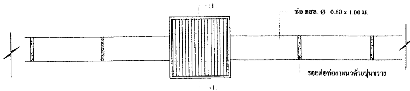
แปลนบ่อพัก.ณ 2133ทอ SCALE: NO SCALE
