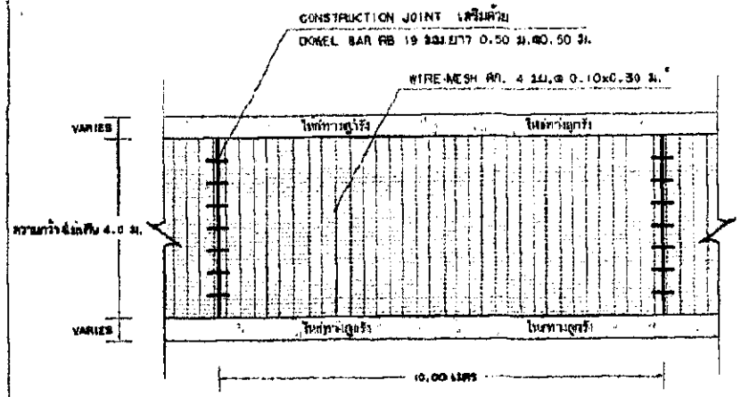
รูปแปลนผิววางรอยคอนกรีตเสริมเหล็ก SCALE: NOT
