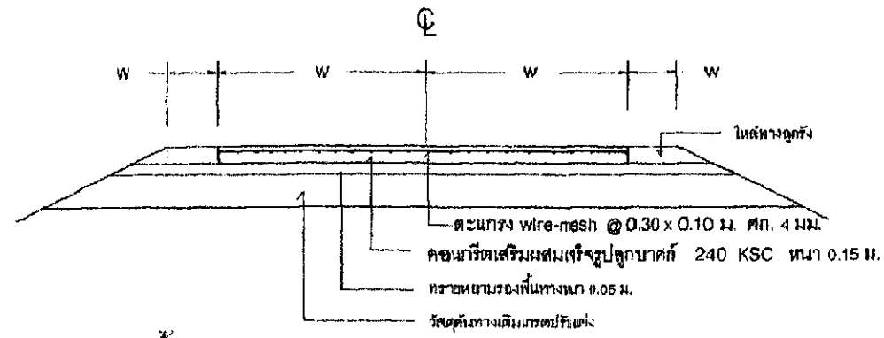
รูปตัดตามรอยคอนกรีตเสริมเหล็ก SCALE: NOT
