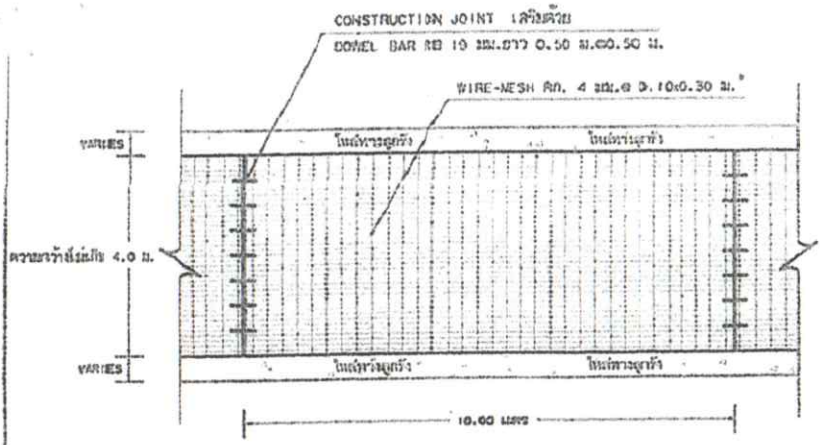
รูปแบบสันผิวจราจรคอนกรีตเสริมเหล็ก SCALE NOT
