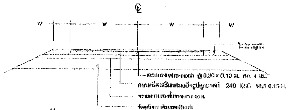
รูป 4. โครงสร้างของคอนกรีตเสริมเหล็ก SCALE: 1/10
