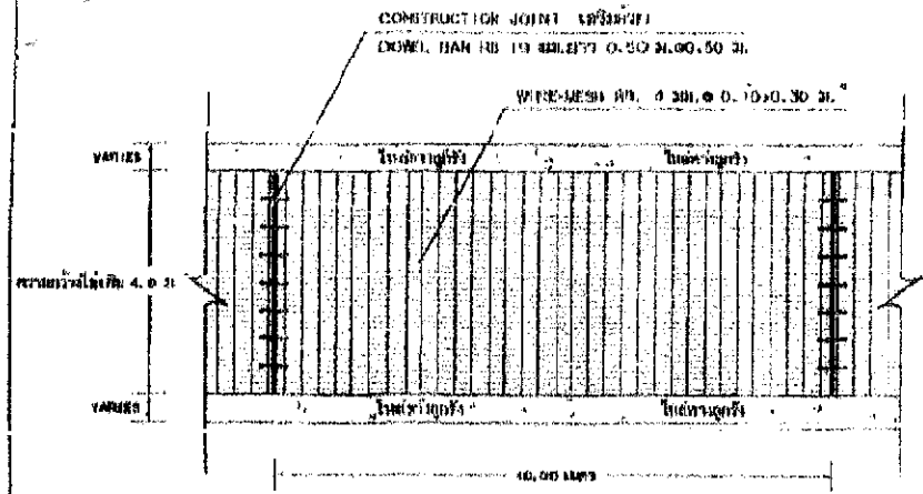
รูป 1. โครงสร้างของคอนกรีตเสริมเหล็ก SCALE: 1/10
