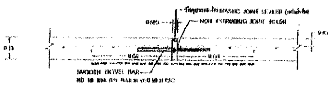
รูป 2. โครงสร้างของ EXPANSION JOINT ทุกกระยะ 50 ซม. SCALE: 1/10
