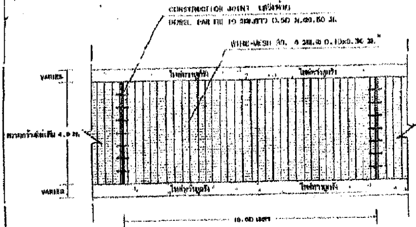
รูปแปลนค้ำยันของคอนกรีตเสริมเหล็ก SCALE: _____
