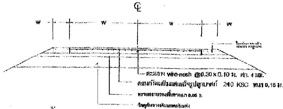
รูปตัดตามแนวของค้ำยันเสริมเหล็ก SCALE: _____
