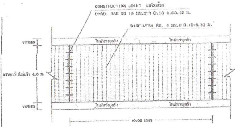
รูปแบบเสริมด้วยจากรองเสริมเหล็ก SCALE: NOT
