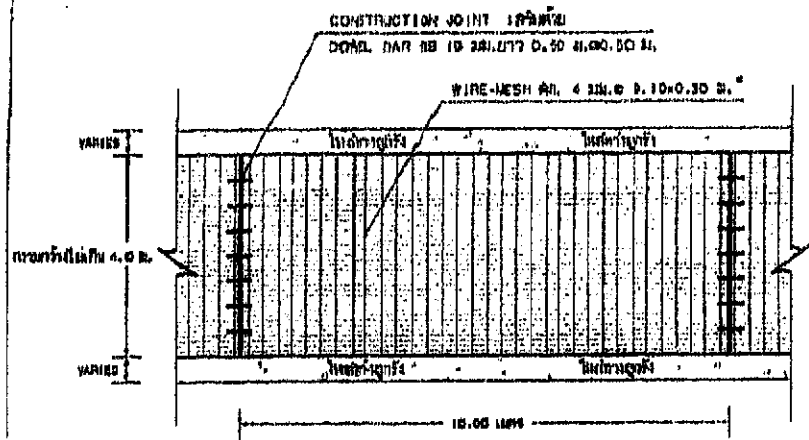
รูปแปลนผิววางจอยคานกรีตเสริมเหล็ก SCALE: NOT
