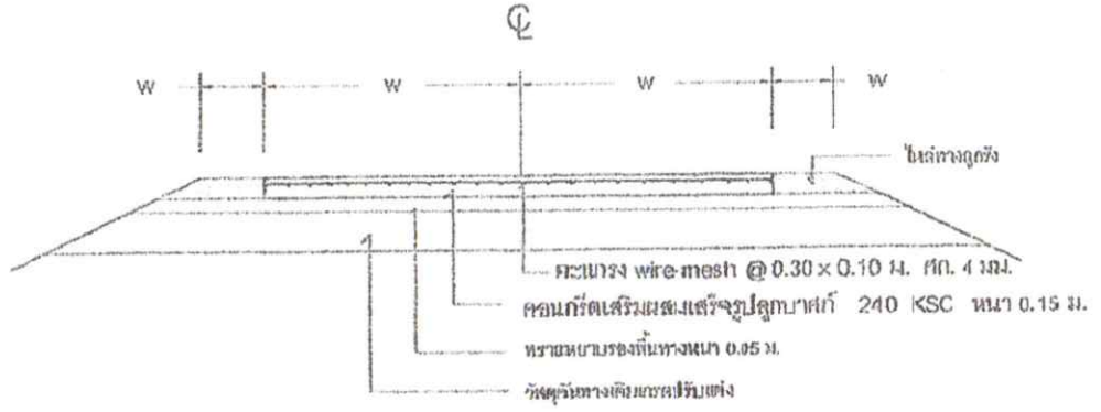
รูปแบบถนนคอนกรีตเสริมเหล็ก SCALE: 1:10
