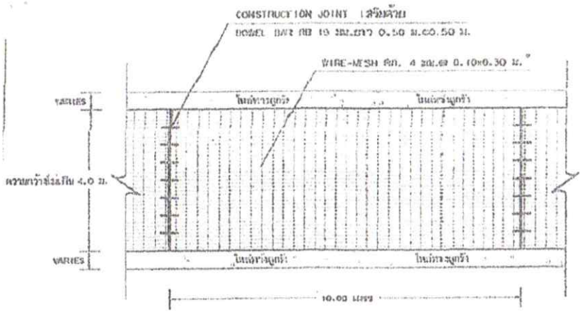
รูปแบบผิวจราจรคอนกรีตเสริมเหล็ก SCALE: 1:30
