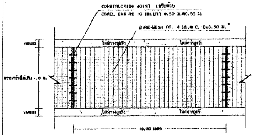
รูปแปลนผิวจราจรคอนกรีตเสริมเหล็ก SCALE 1:20
