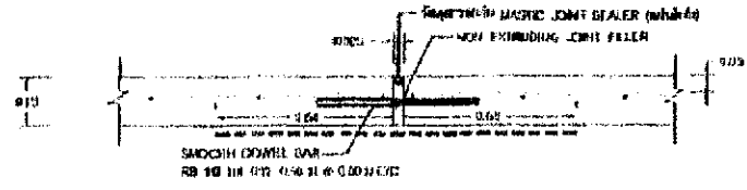
ขนาดของข้อ EXPANSION JOINT ทุกระยะ 50 เมตร SCALE 1:20
