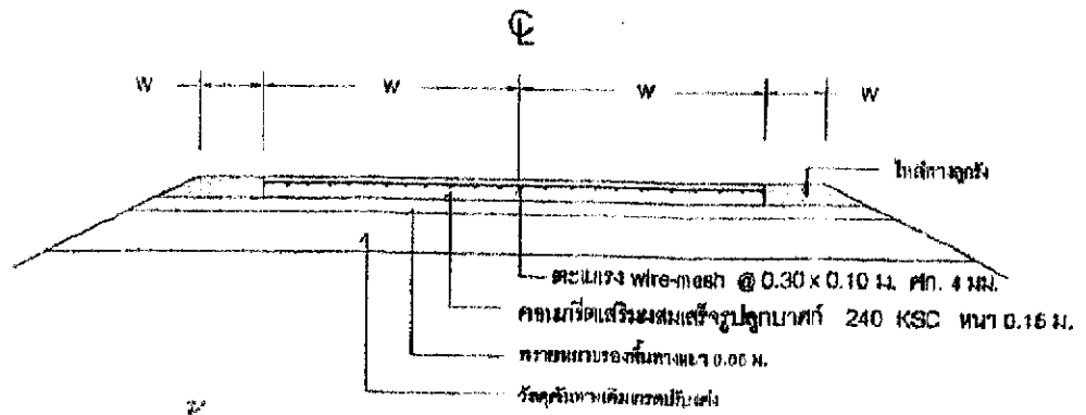
รูปตัดถนนคอนกรีตเสริมเหล็ก SCALE 1:20
