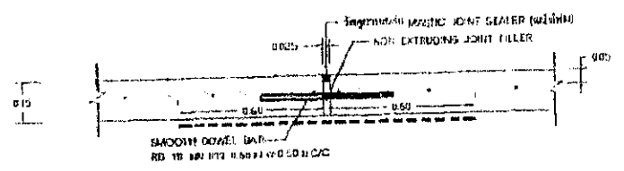
รายละเอียด EXPANSION JOINT ทุกระยะ 50 เมตร SCALE: NOT
