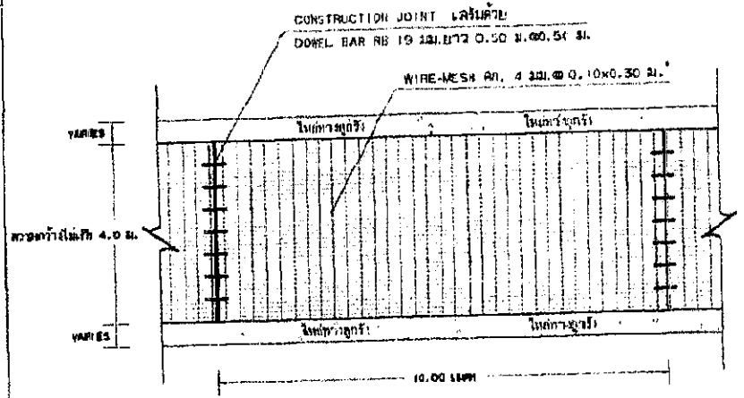
รูปแบบฉนวนผิวจราจรคอนกรีตเสริมเหล็ก SCALE: NOT
