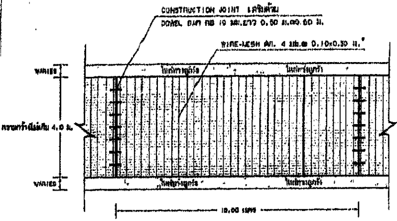
รูปแปลนผิววางคอนกรีตเสริมเหล็ก SCALE: NOT
