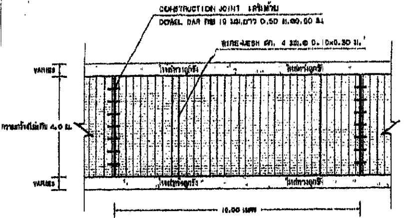
รูปแบบผนังของคอนกรีตเสริมเหล็ก SCALE ..... NOT
