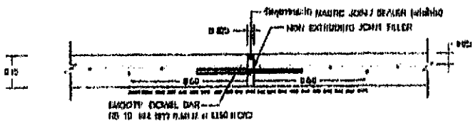
ขยายของผนัง EXPANSION JOINT ทุกระยะ 50 ซม. SCALE ..... NOT
