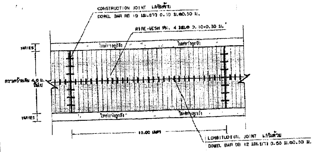
รูปแปลนผิวจราจรคอนกรีตเสริมเหล็ก SCALE _____ NOT
