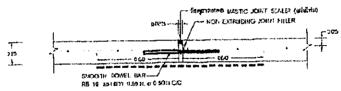
ขยายรอยต่อ EXPANSION JOINT ทุกระยะ 50 เมตร SCALE NOT
