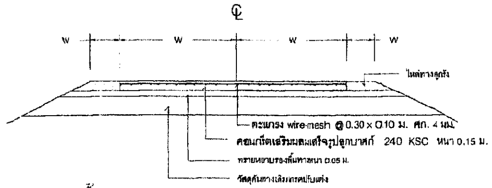
รูปตัดตามคอนกรีตเสริมเหล็ก SCALE NOT
