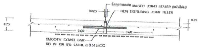
ขยายรอยต่อ EXPANSION JOINT ทุกๆระยะ 50 เมตร SCALE _____ NOT
