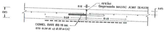
ขยายรอยต่อ CONSTRUCTION JOINT ทุกๆระยะ 10 เมตร SCALE _____ NOT
