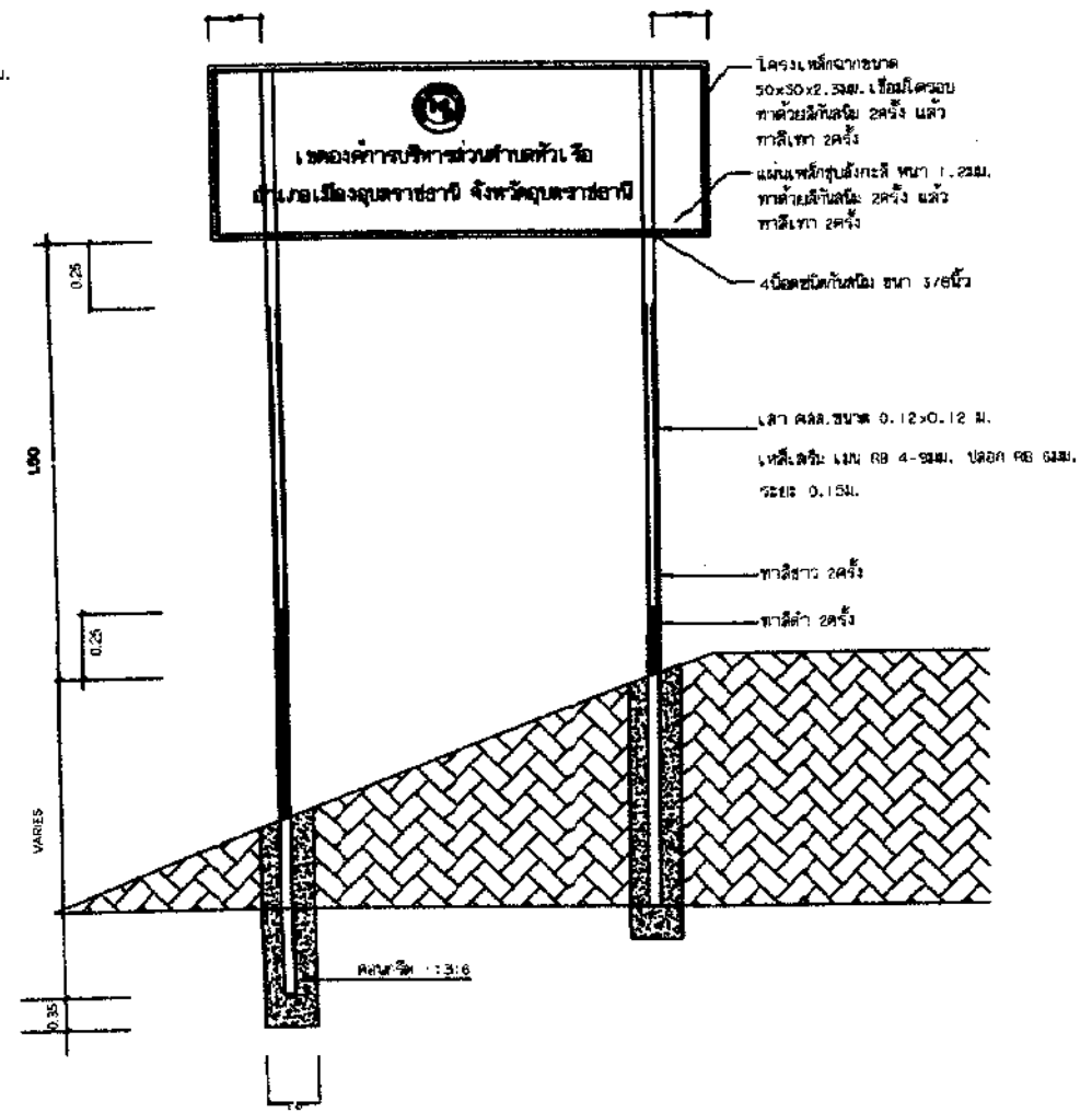
แสดงรายละเอียดโครงสร้างป้ายและวิธีการปักป้าย
