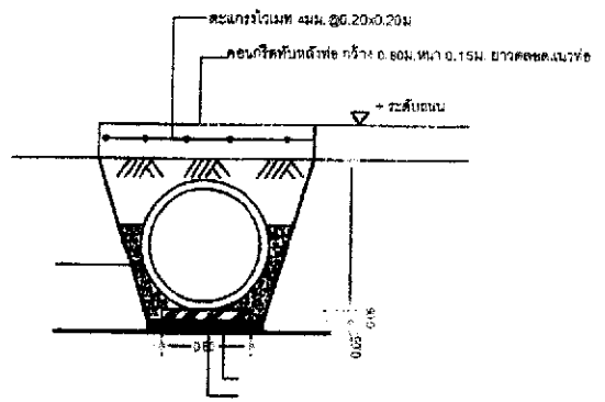
รูปตัดแนววางท่อ
