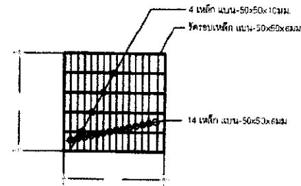
รูปขยายเหล็กฝาดตะแกรงบ่อพัก
