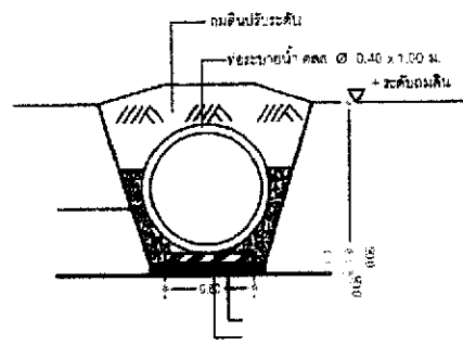
รูปตัดแนววางท่อ
