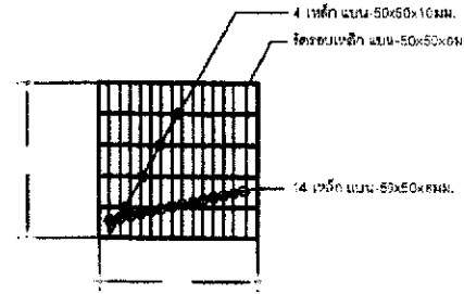
รูปขยายเหล็กฝาดะแกรงบ่อพัก
