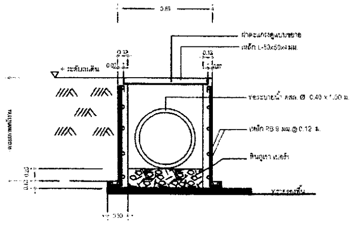
รูปตัดบ่อพักแบบธนาคารน้ำ
