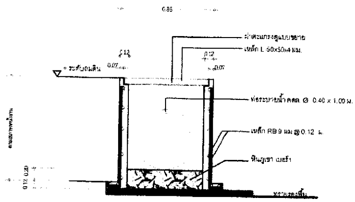
รูปตัดบ่อพักแบบธนาคารน้ำ
