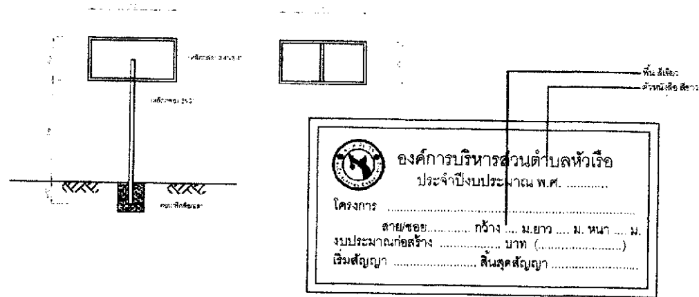
รายละเอียดประกอบ แบบป้ายมาตรฐานสำหรับโครงการขององค์การบริหารส่วนตำบล
